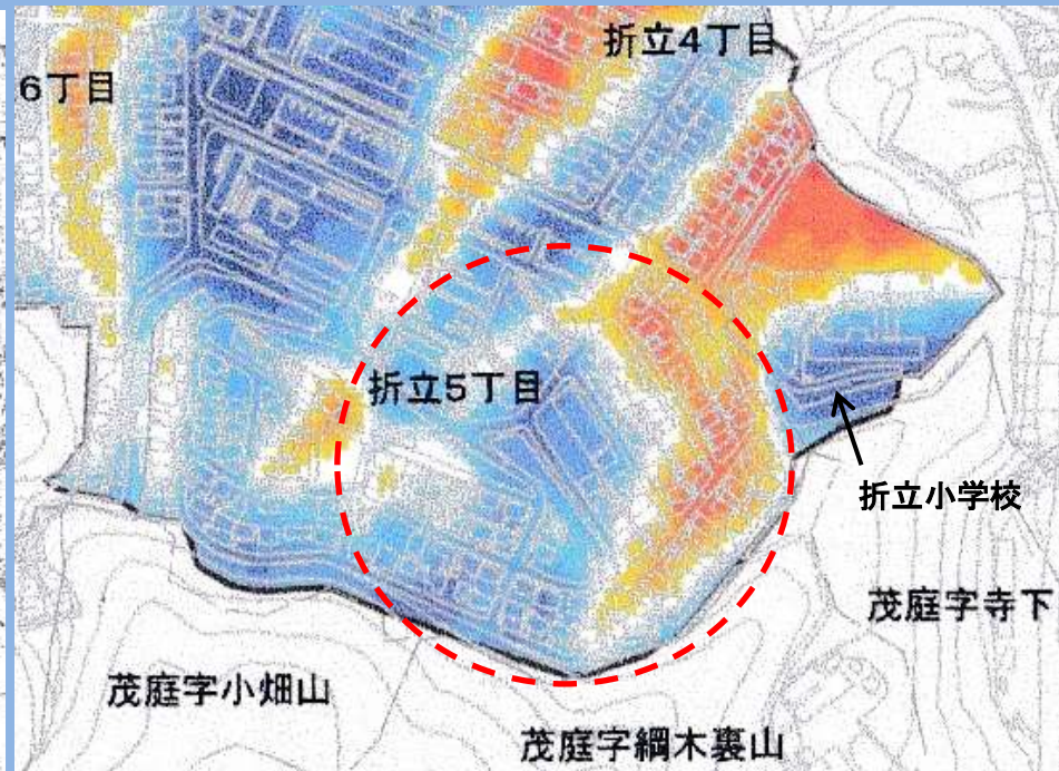
切土・盛土図
